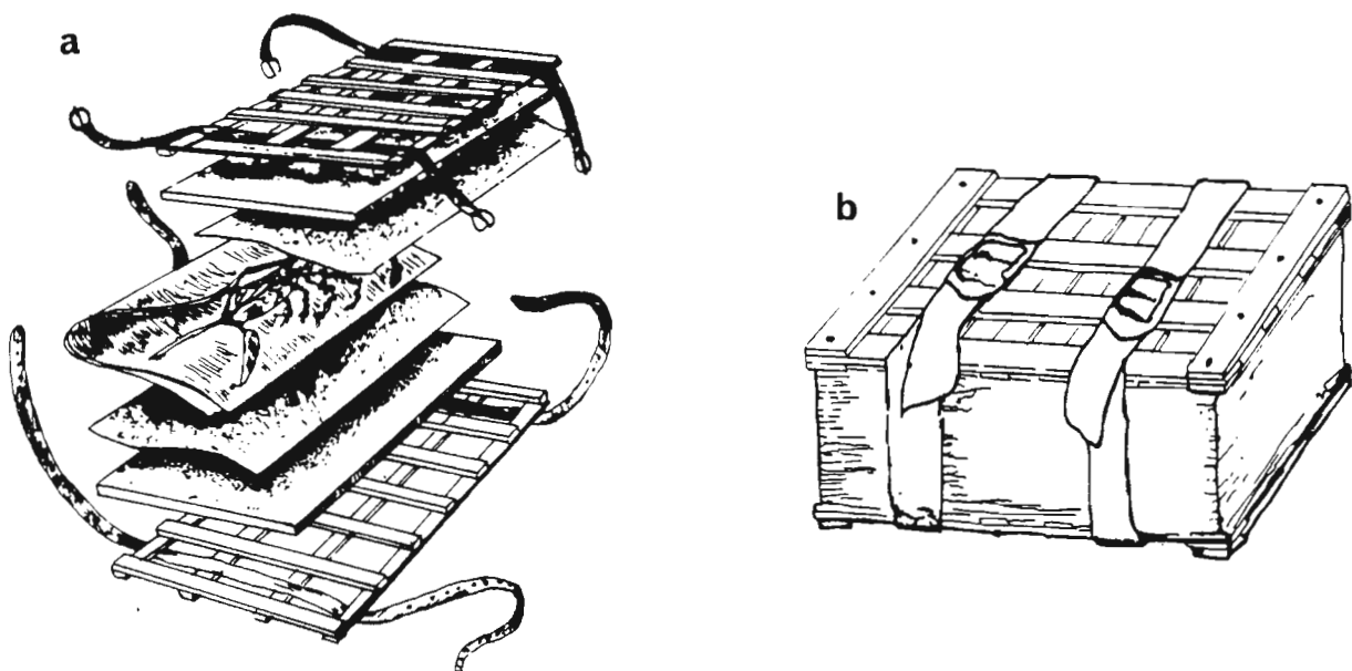
Figura 2 a. Partes de una prensa. b. Prensa construida.
