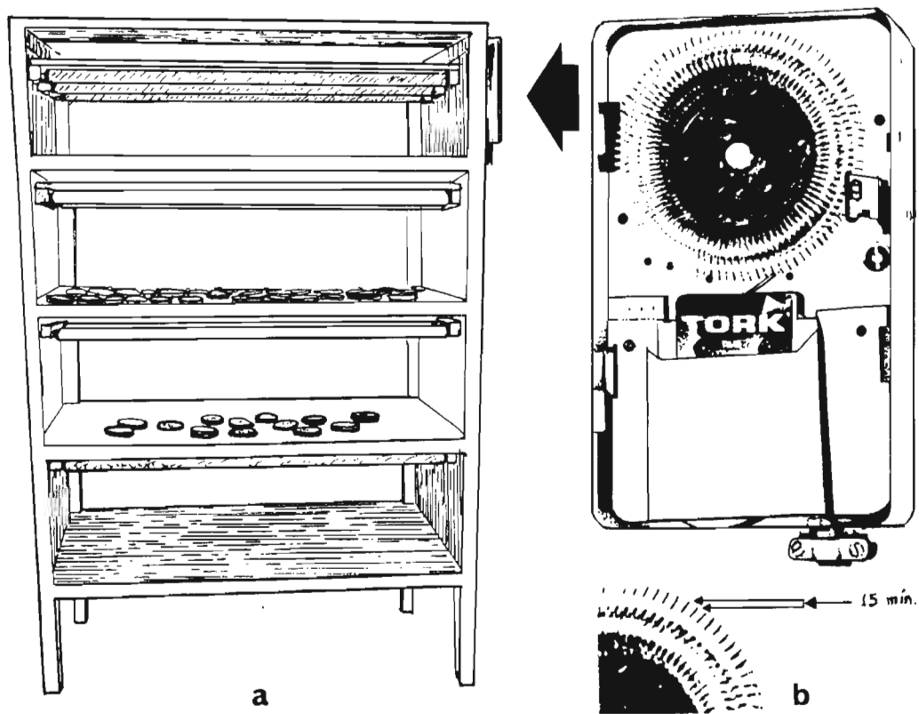
Figura 3 a. Cámara de crecimiento de construcción artesanal. b. Reloj control para regular la iluminación.
