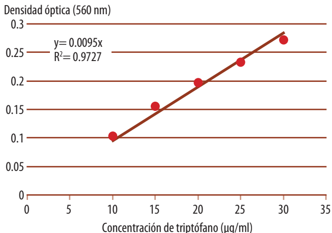
Apéndice: Figura 1. Ejemplo de una curva de calibración para el triptófano.
