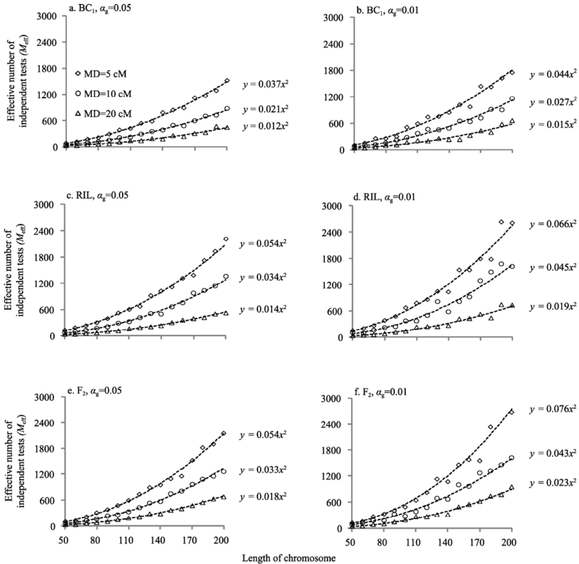
图 4 定位上位性互作 QTL 的二维扫描中不同标记密度下有效独立检验次数( M_{eff} )与染色体长度(CL)呈二次幂关系
