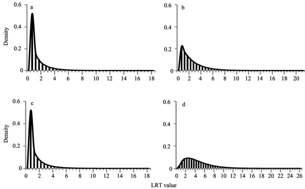
图 1 一维和二维 QTL 作图扫描过程中单个扫描位点 LRT 统计量与卡方分布的拟合
