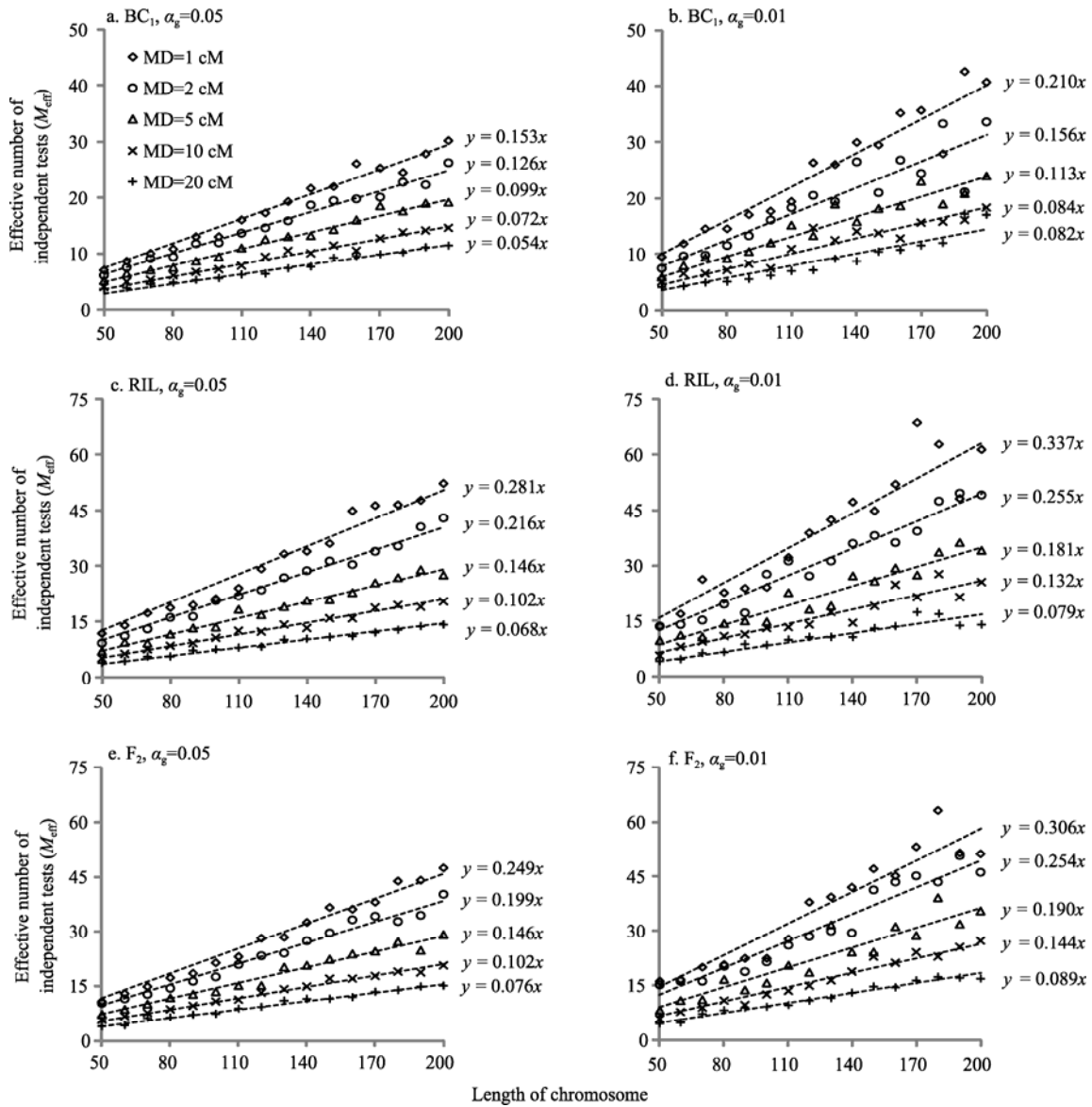
图 3 定位加显性效应 QTL 的一维扫描中不同标记密度下有效独立检验次数( M_{eff} )与染色体长度(CL)呈线性关系
